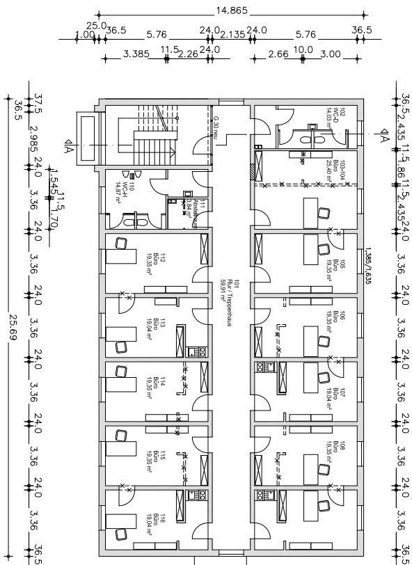
Grundriss Obergeschoss
