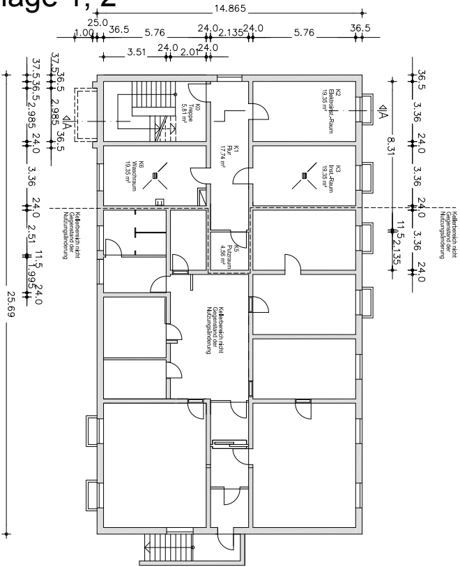
Grundriss Kellergeschoss
