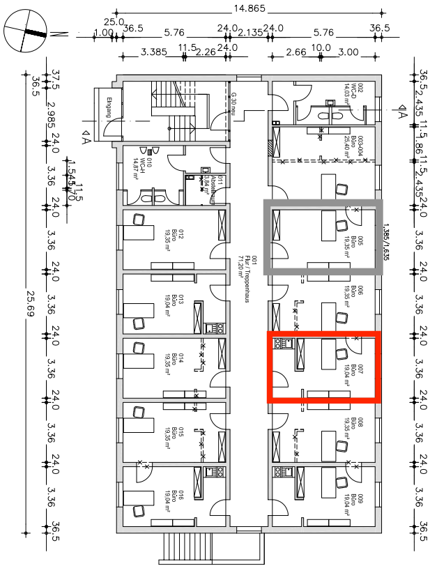
Grundriss Erdgeschoss
